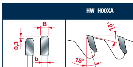
Форма зуба
